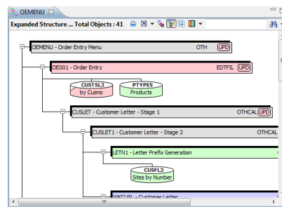
Diagrammes de structures des programmes
